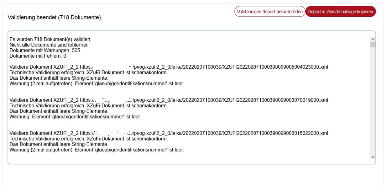
Abbildung 6: Validierungsfehler
